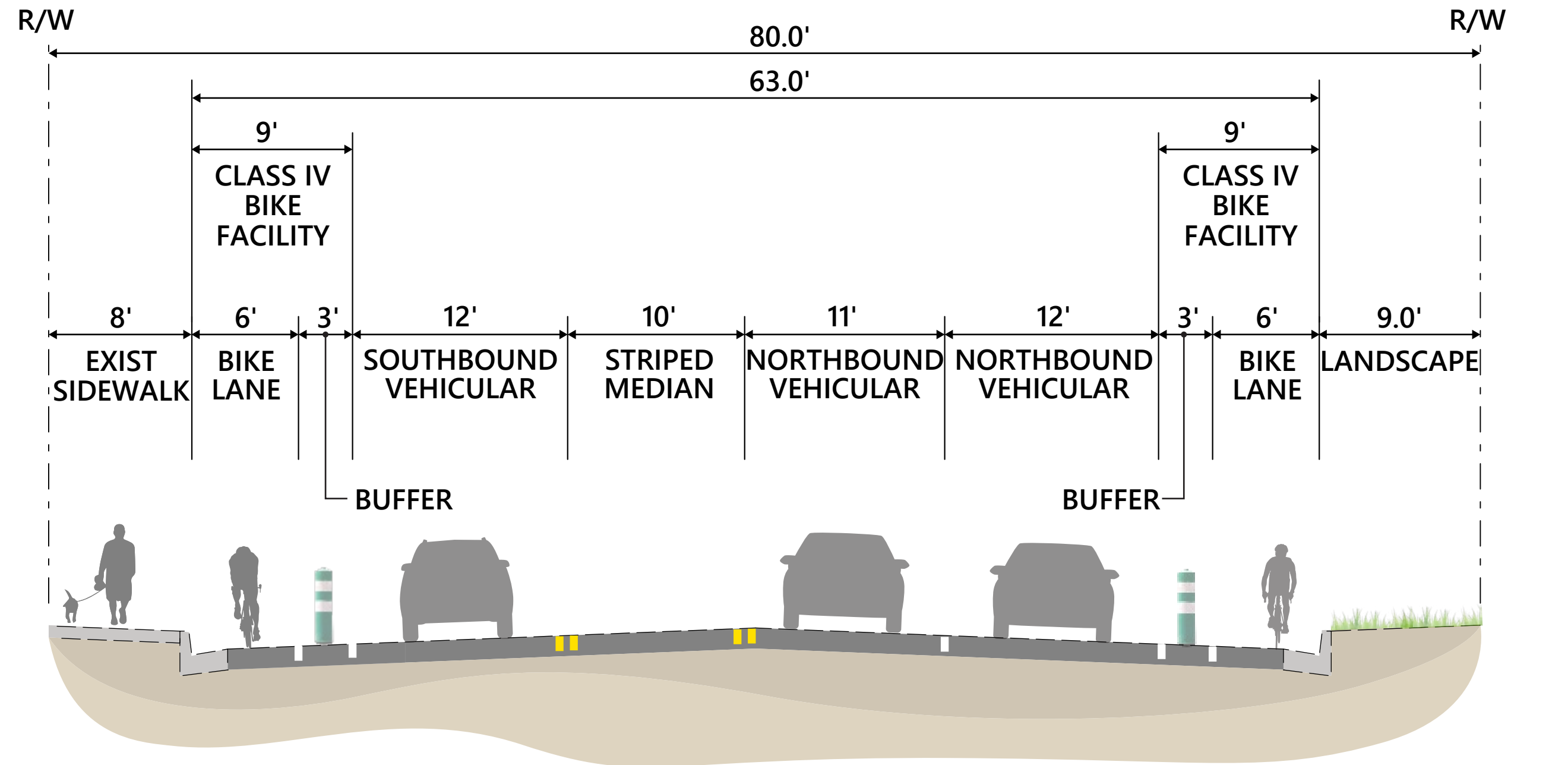
SECTION D-D
