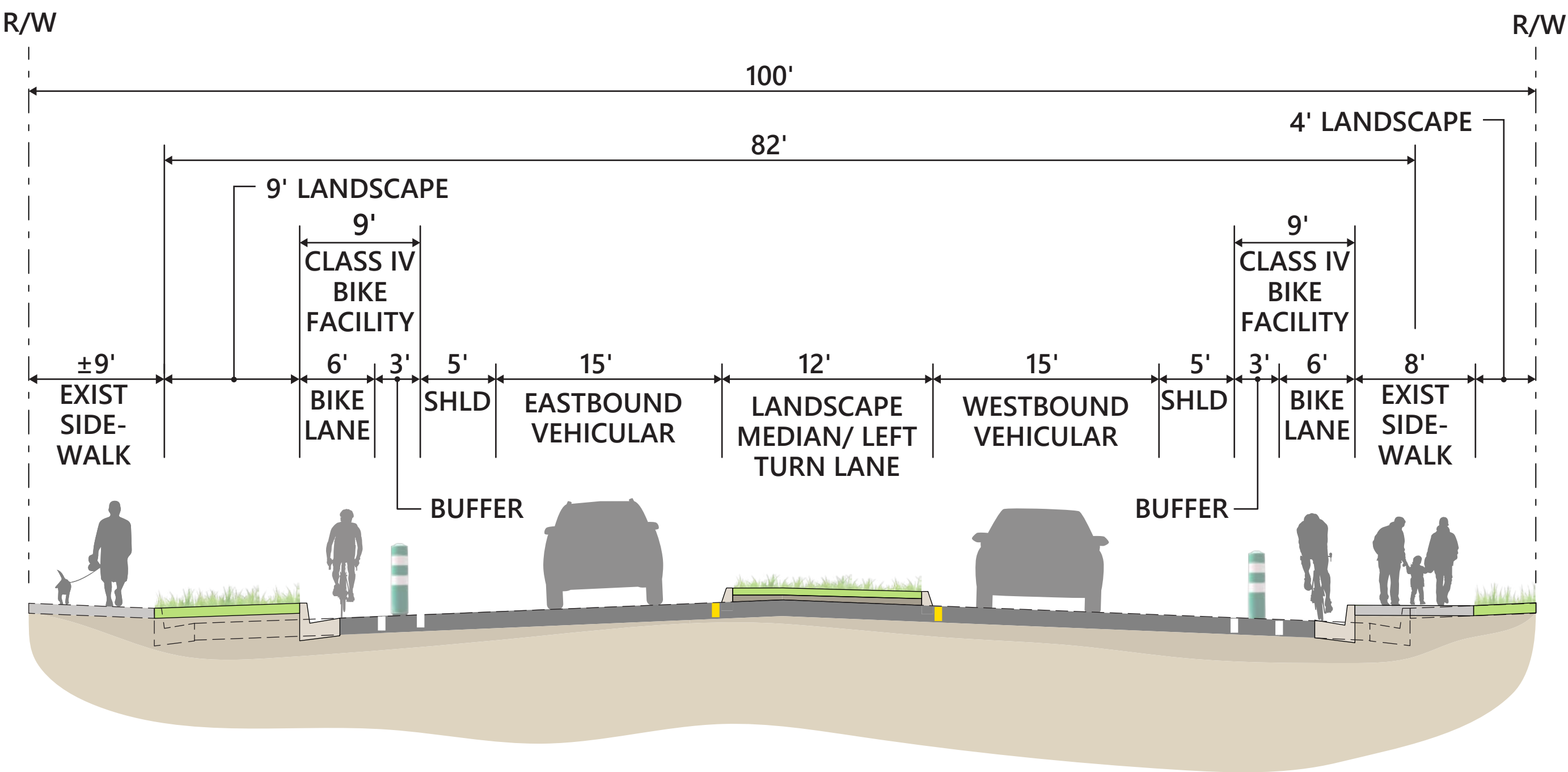
SECTION A-A
